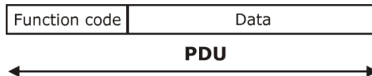
Рисунок 4: Состав PDU
