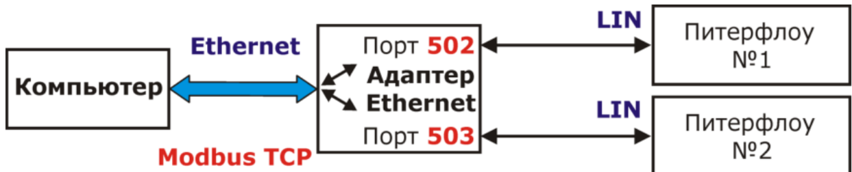
Рисунок 1: Адаптер Ethernet↔Прибор
