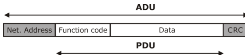
Рисунок 5: ADU для «Modbus RTU»
