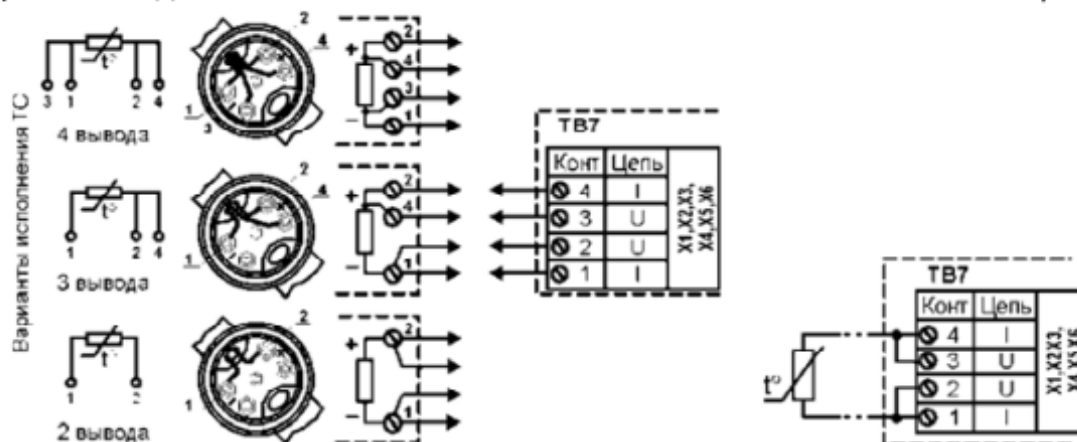
Рис. 4.2 - Варианты подключения ТС
