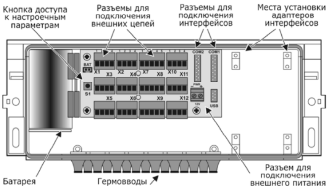
Рис. 2.2 – Вид на монтажный отсек при снятой крышке
