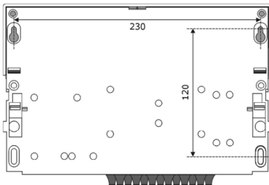
Рис. 4.1 – Схема крепления корпуса ТВ7
