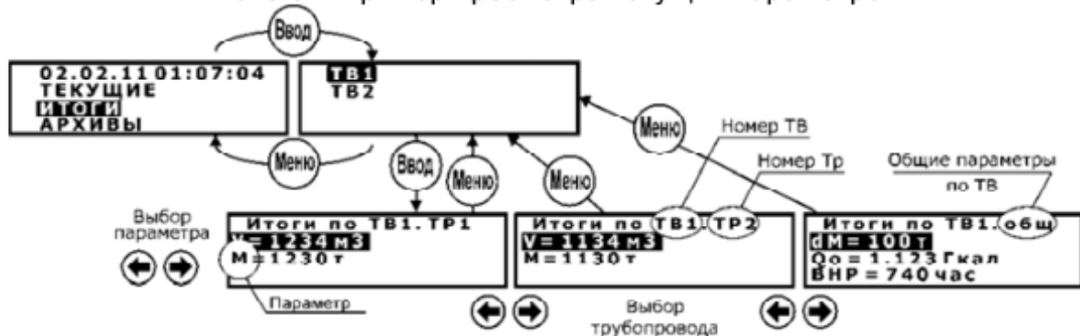
Рис. 3.4 – Пример просмотра итоговых параметров
