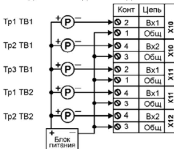
Рис. 4.4 – Пример подключения датчиков давления
