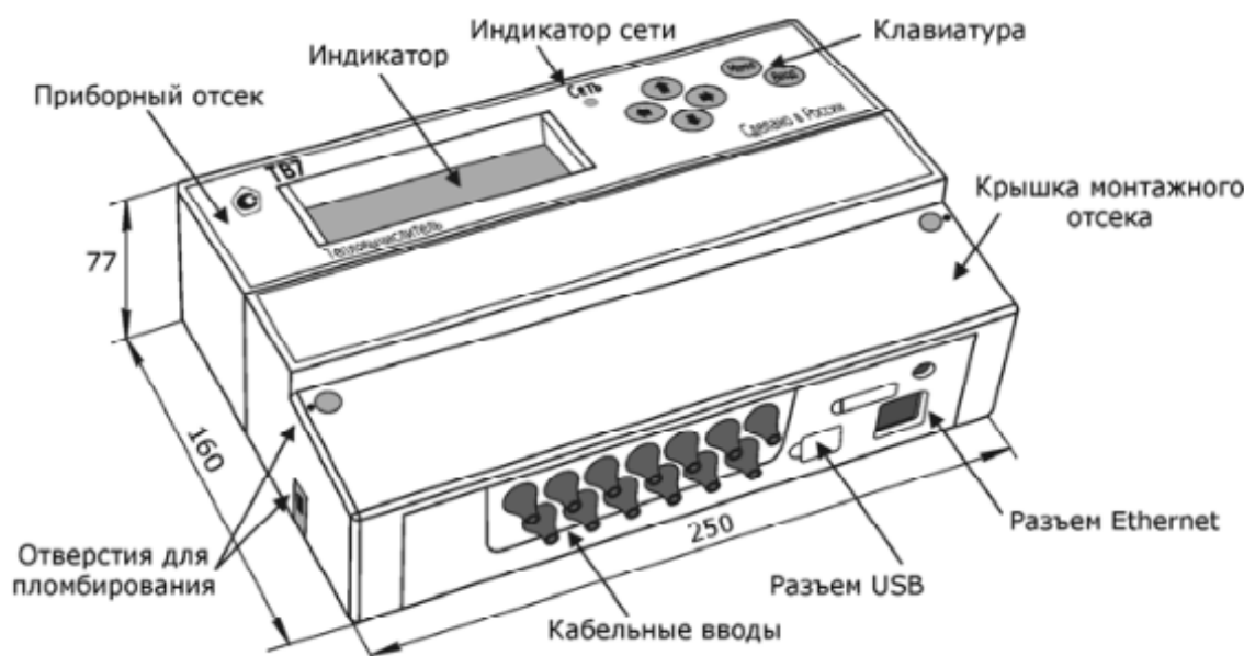
Рис. 2.1 – Внешний вид ТВ7
