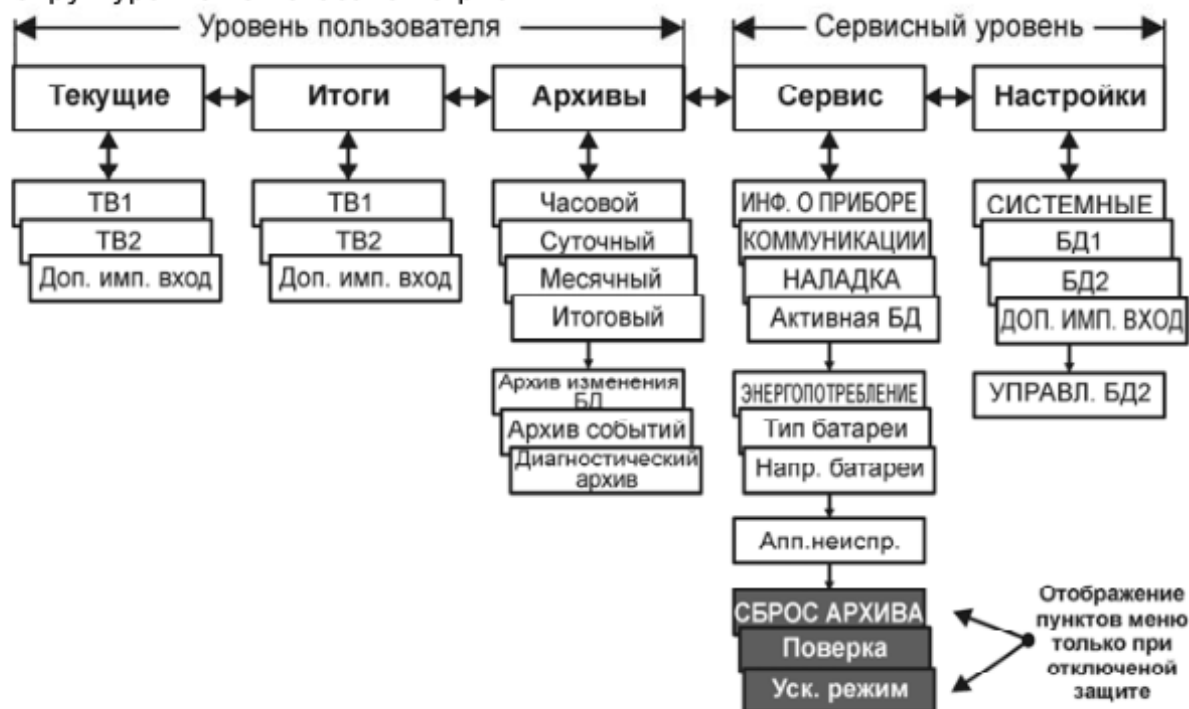
Рис. 2.1 – Структура меню тепловычислителя
