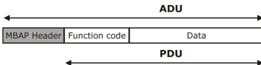
Рисунок 4: ADU для «Modbus TCP»
