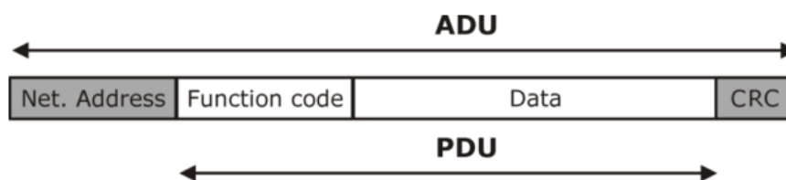
Рисунок 3: ADU для «Modbus RTU»
