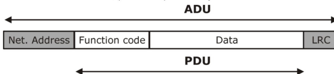
Рисунок 2: ADU для «Modbus RTU/ASCII»
