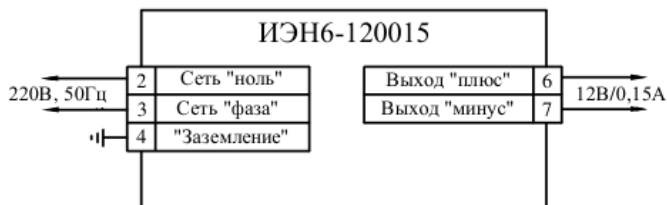
Рис. 2 Схема подключения
