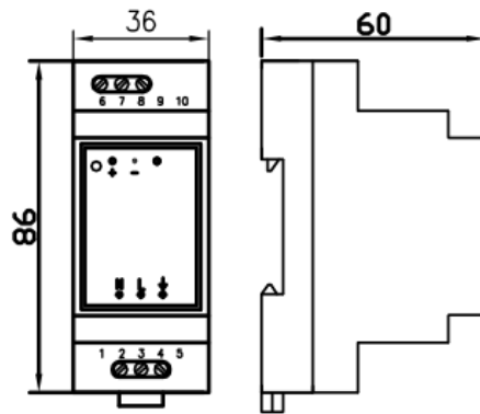
Рис. 1 - Габаритный чертеж
